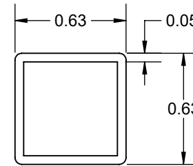
SQ BALUSTER
